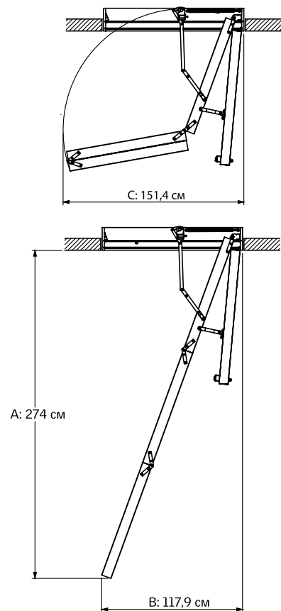
Чертеж чердачной лестницы «Престиж»
